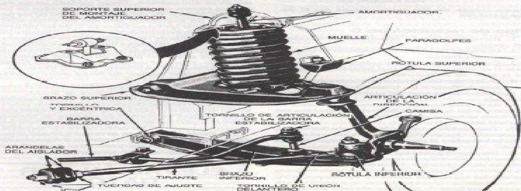
Suspensión delantera. Muelle sobre el brazo superior
