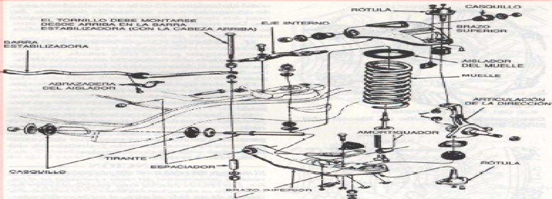
Suspensión delantera. Muelle y brazo inferior
